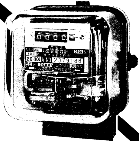
OBOG型広範囲单相積算電力計
